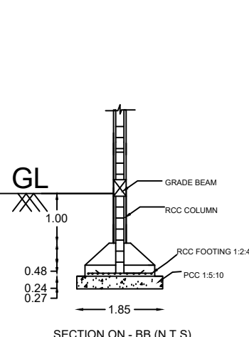
SECTION ON - BB (N.T.S)
