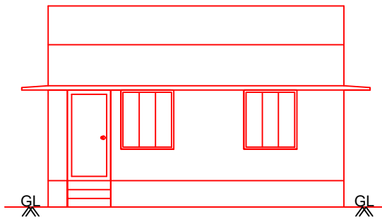
ELEVATION
