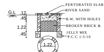
R.W.C.T, PLAN & SECTION
