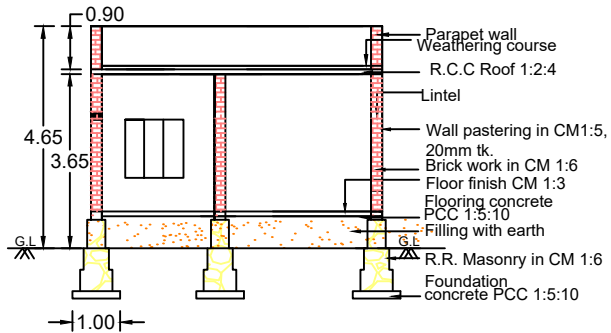
SECTION A-B
