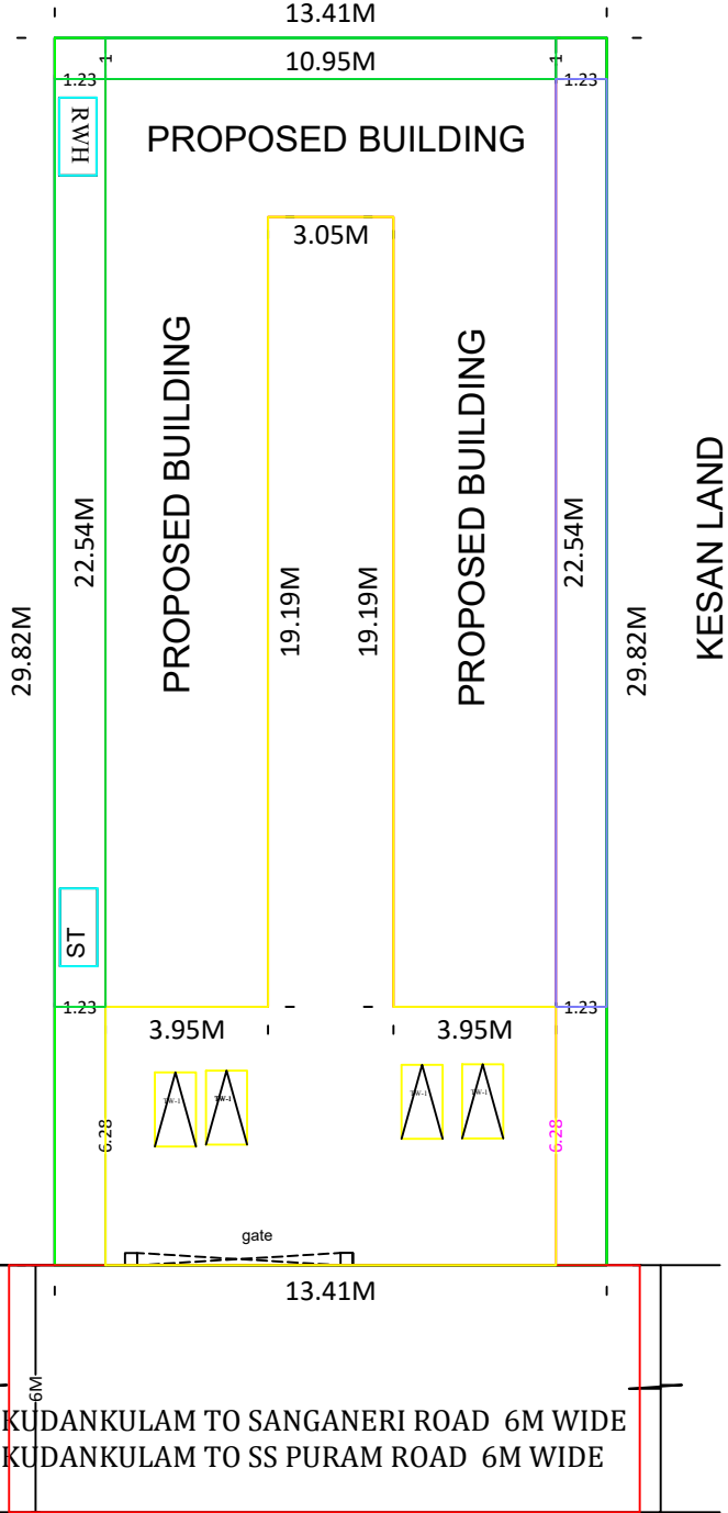
SITE PLAN 1:100 SCALE
