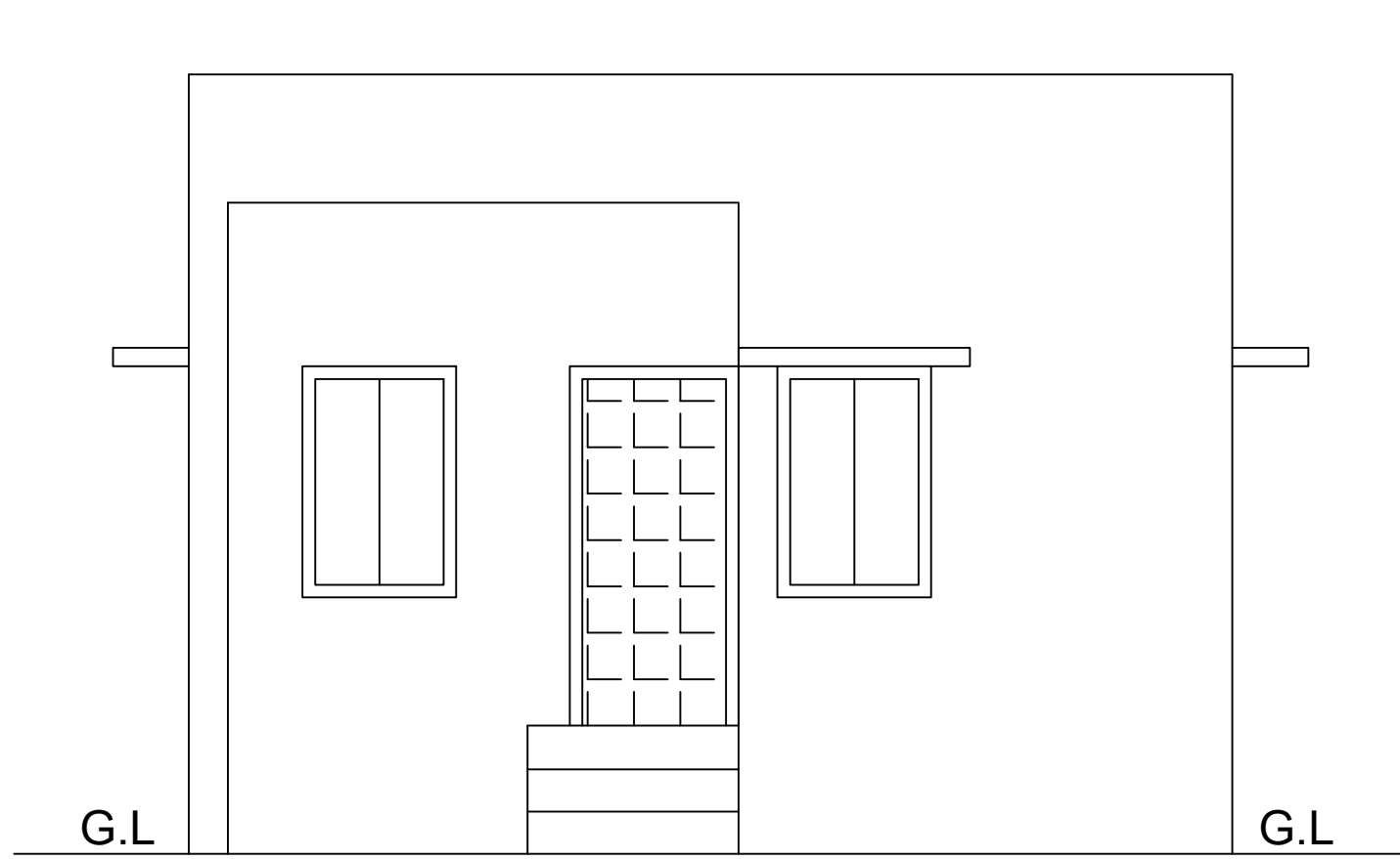
ELEVATION
