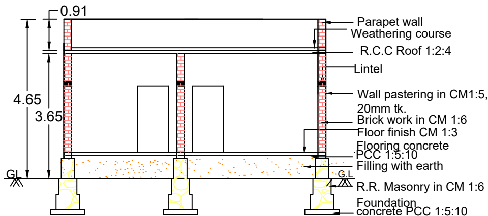
SECTION A-B
