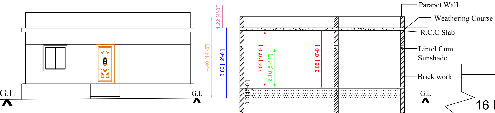
ELEVATION
