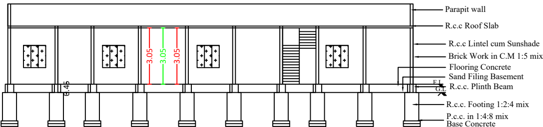
SECTION A-B
