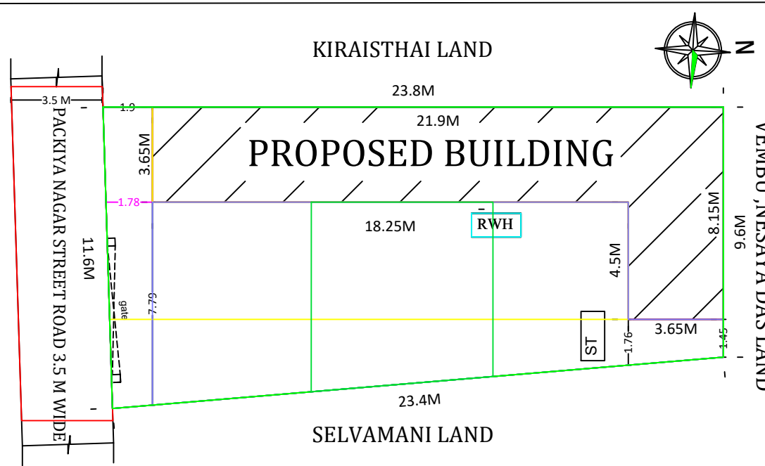
SITE PLAN 1:100 SCALE
