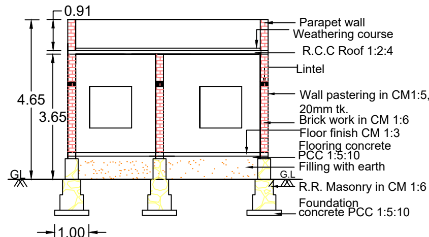
SECTION A-B
