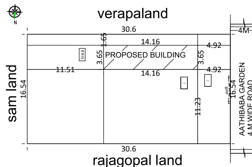
SITE PLAN 1:100 SCALE
