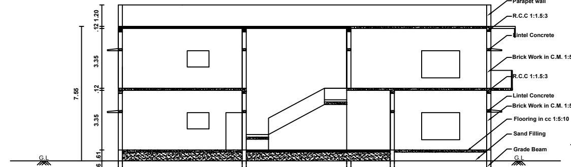
SECTION 'AB'
