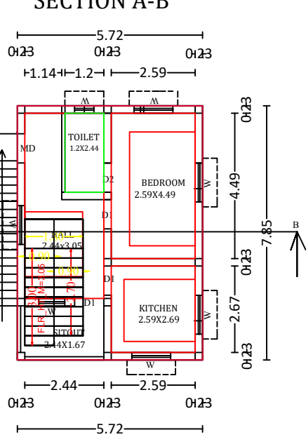
F.F. PLAN
