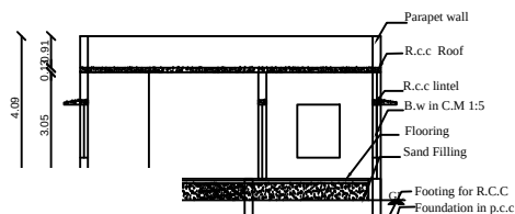
SECTION A&amp;B
