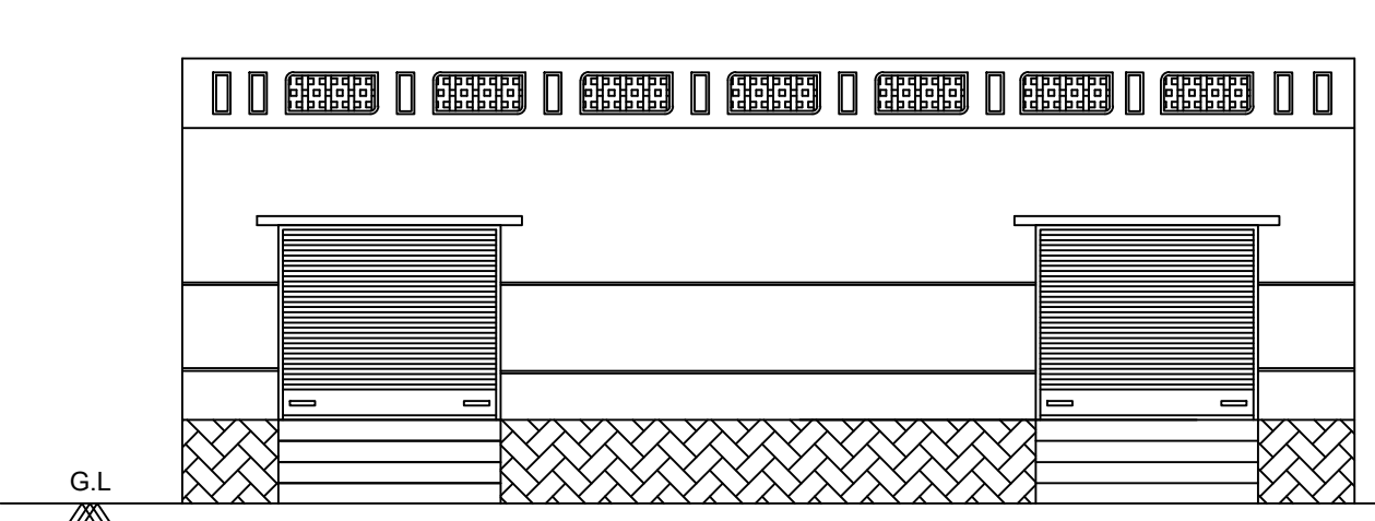
ELEVATION
