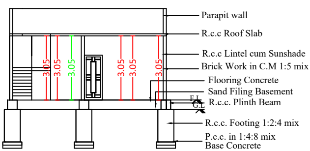
SECTION A-B
