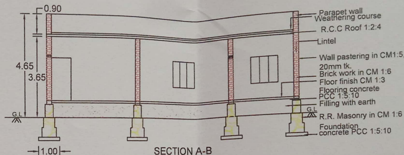
SECTION A-B
