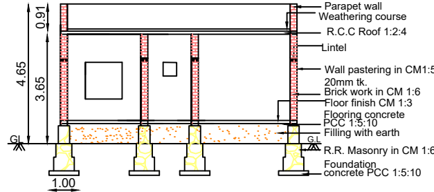
SECTION A-B
