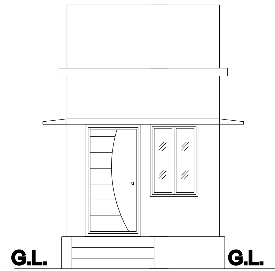
ELEVATION
