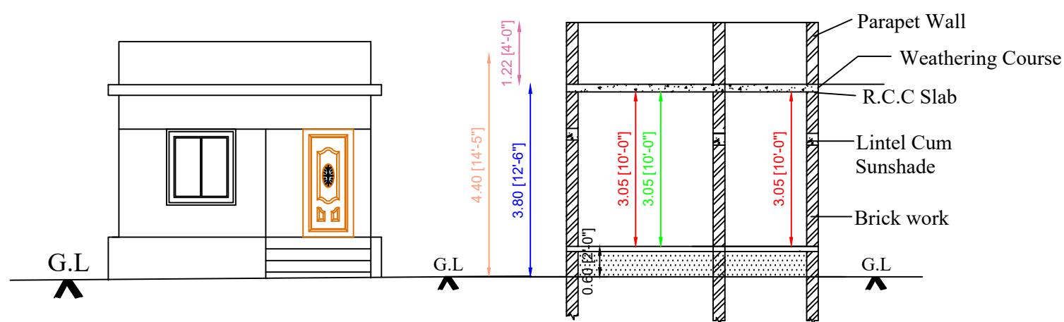
ELEVATION
