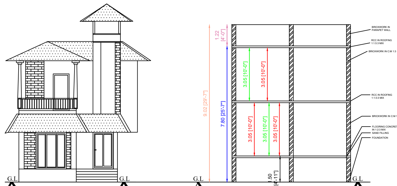
ELEVATION
