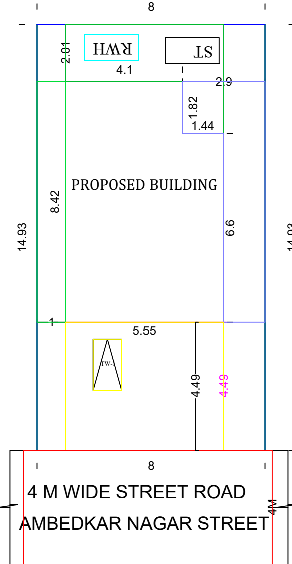
SITE PLAN 1:100 SCALE
