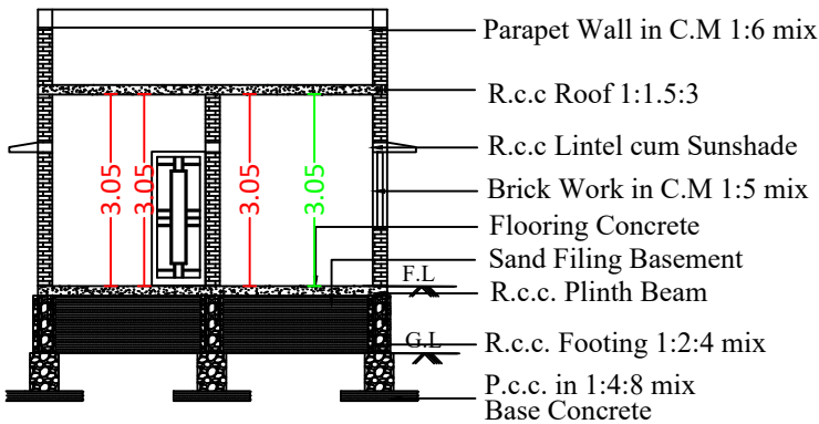
SECTION A-B
