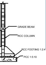
SECTION ON - BB (N.T.S)
