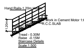
Staircase Details Scale: 1:500
