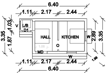
G.F PLAN
