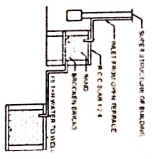
SECTION ON - BB (N.T.S)
