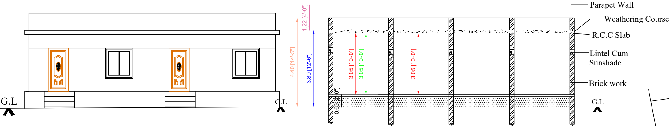
ELEVATION
