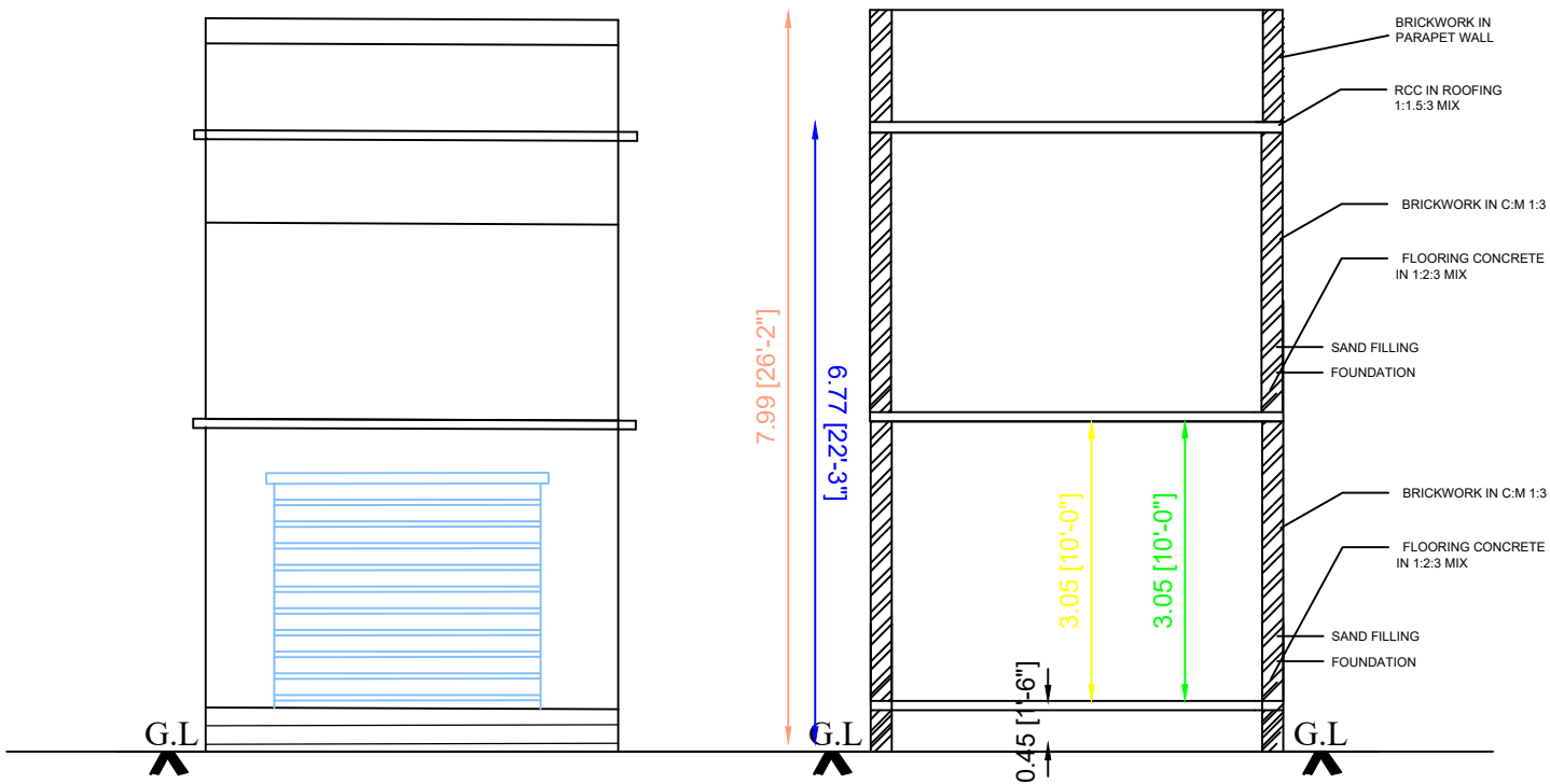
ELEVATION
