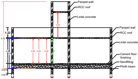
SECTION - AB
