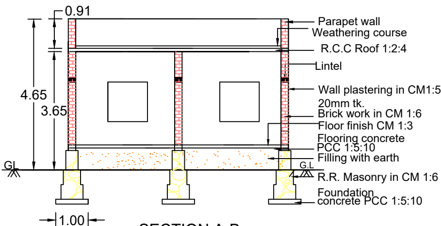
SECTION A-B
