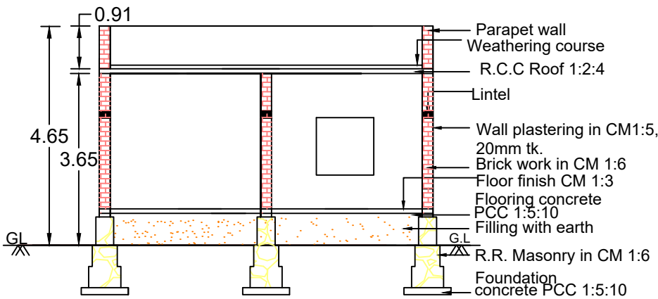
SECTION A-B
