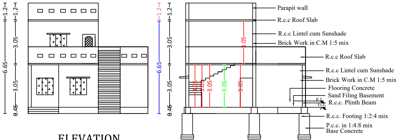
SECTION A-B
