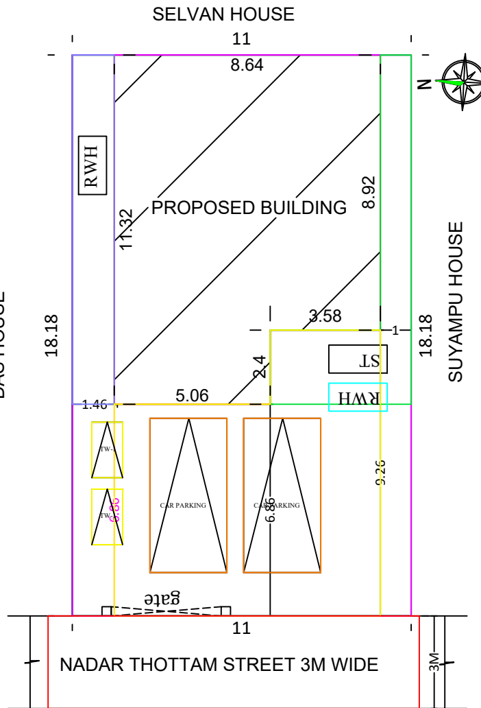
SITE PLAN 1:100 SCALE
