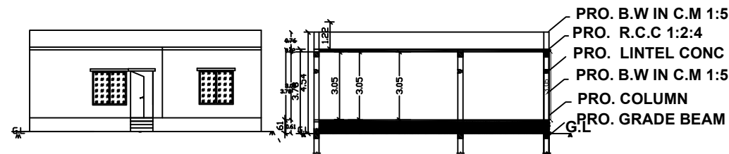
ELEVATION
