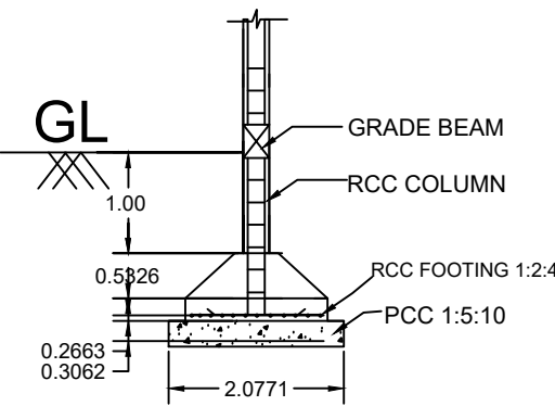
SECTION ON - BB (N.T.S)
