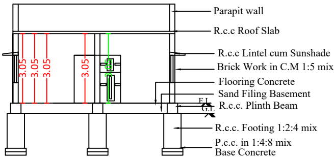
SECTION A-B
