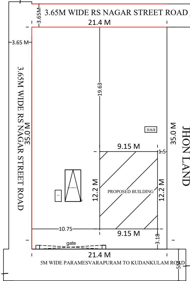
SITE PLAN 1:100 SCALE
