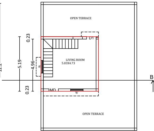
G.F PLAN
