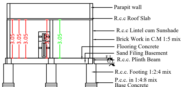
SECTION A-B
