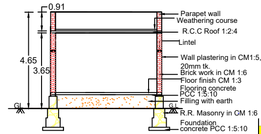
SECTION A-B
