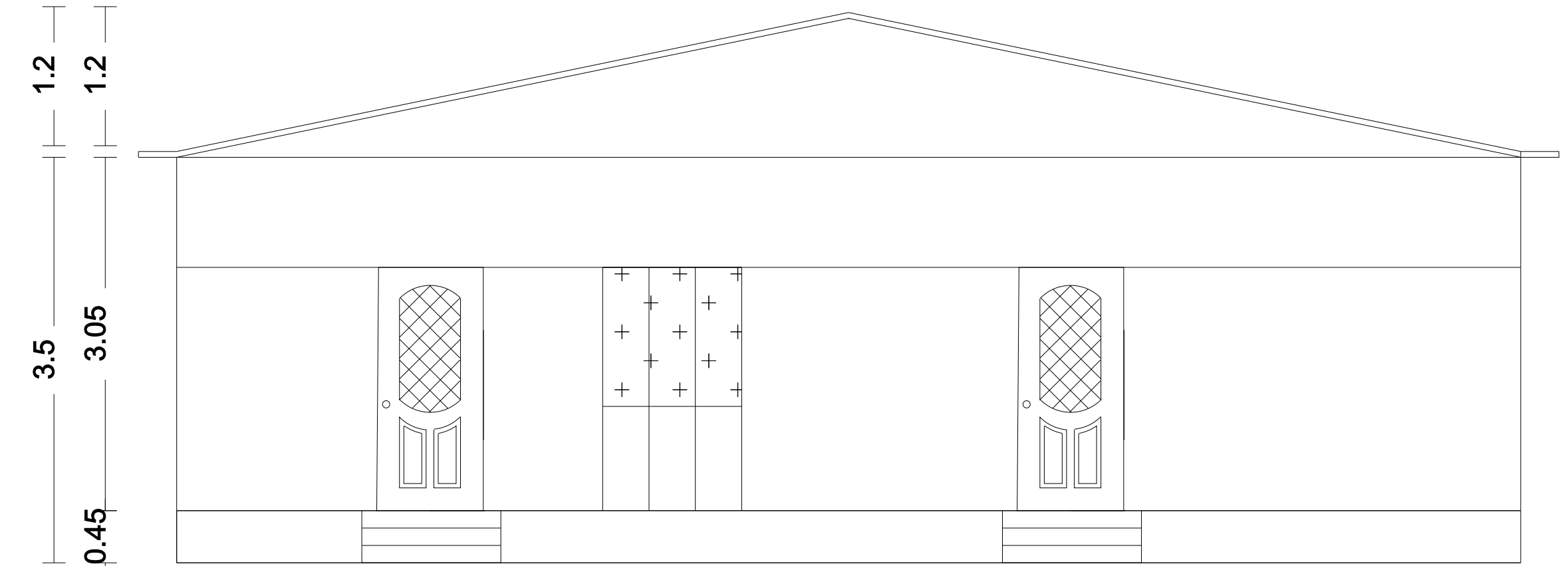
ELEVATION
