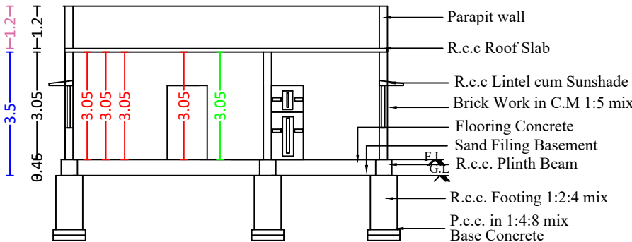
SECTION A-B
