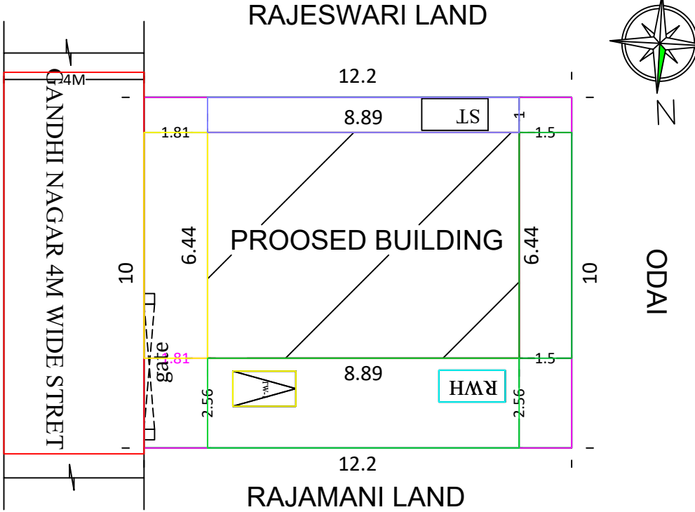
SITE PLAN 1:100 SCALE
