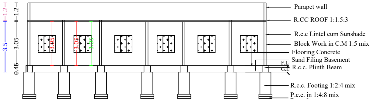
SECTION A-B
