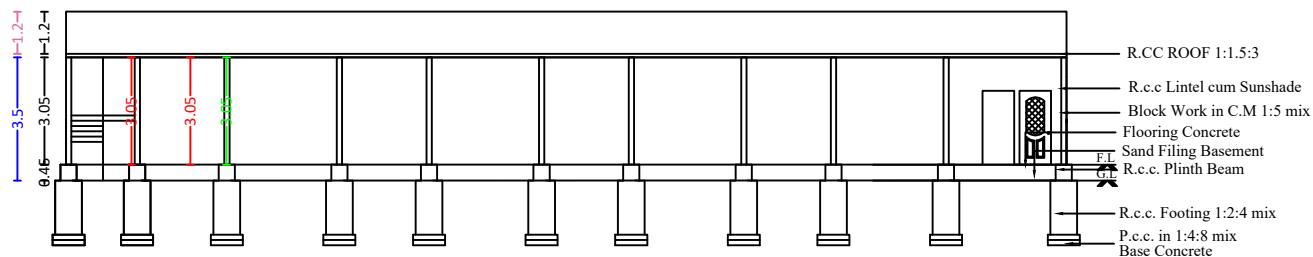
SECTION A-B
