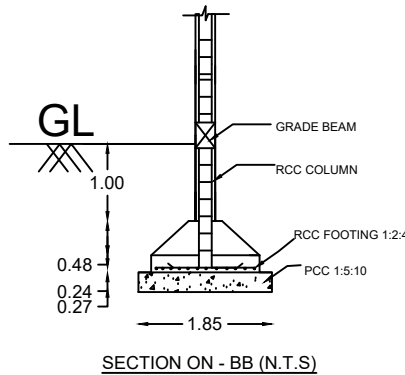
SECTION ON - BB (N.T.S.)
