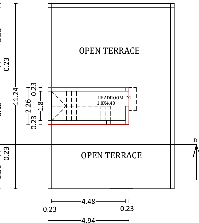
F.F PLAN
