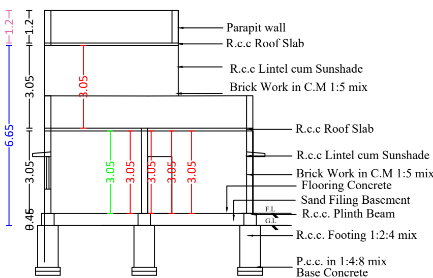
SECTION A-B
