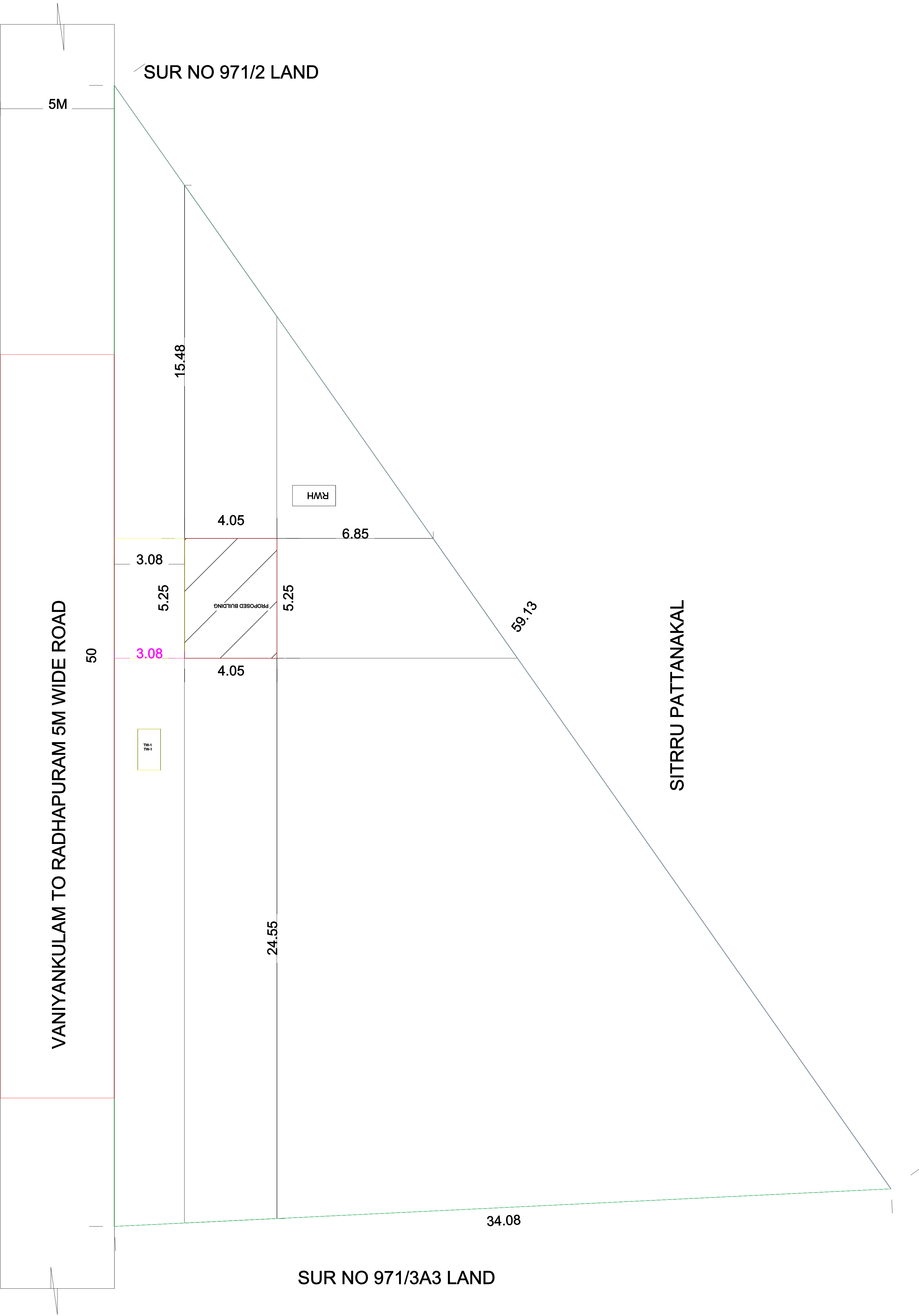
SITE PLAN 1:100 SCALE
