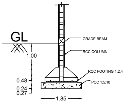
SECTION ON - BB (N.T.S)
