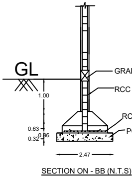
SECTION ON - BB (N.T.S)
