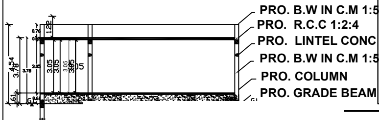
ELEVATION
