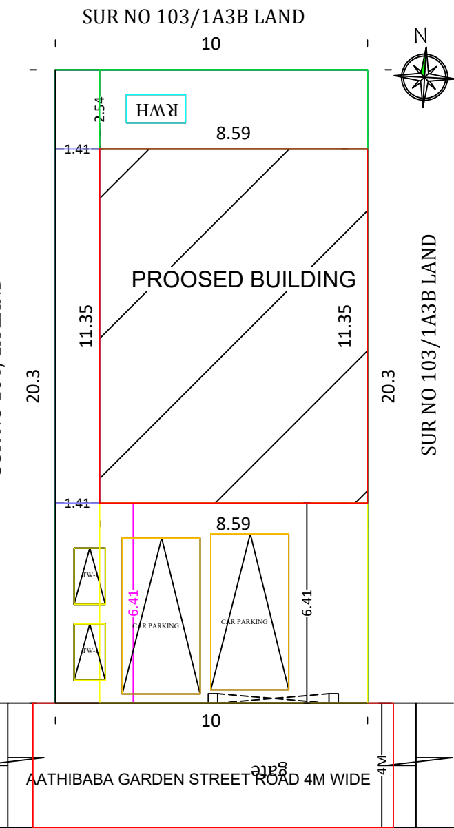
SITE PLAN 1:100 SCALE
