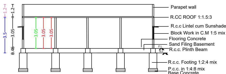
SECTION A-B
