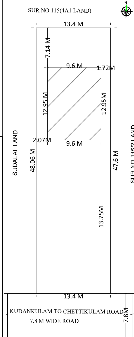
SITE PLAN 1:100 SCALE
